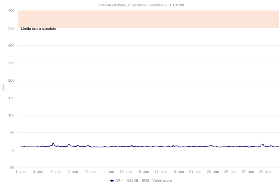
Fig. 1.2.1.1. Concentrațiile medii orare ale poluantului SO 2
