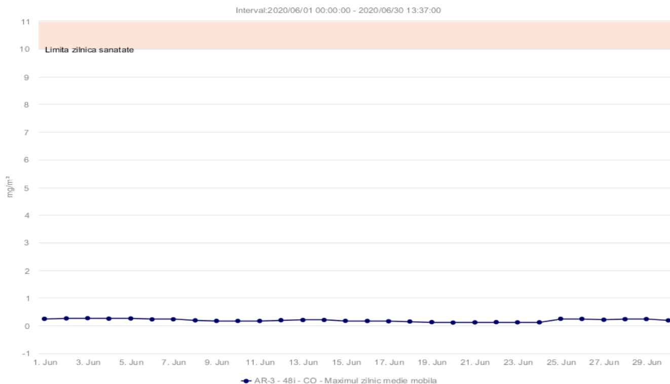
Fig. 1.2.3.3. Concentrațiile medii orare ale poluantului CO
