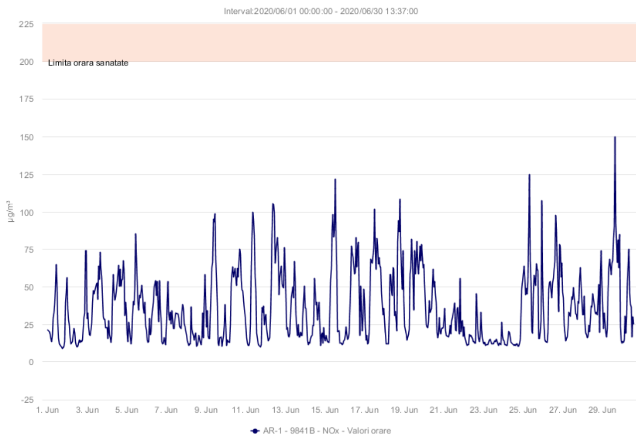
Fig.1.2.2.1. Concentrațiile medii orare ale poluantului \text{NO}_2
