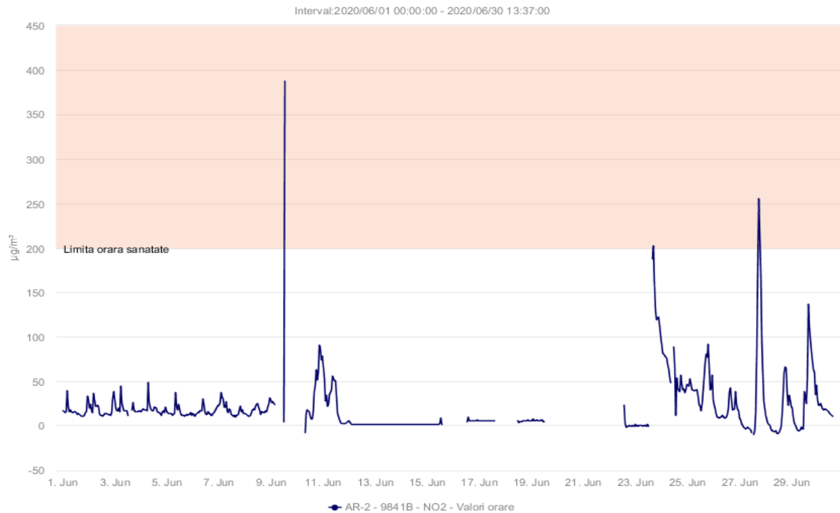
Fig.1.2.2.3. Concentrațiile medii orare ale poluantului NO 2
