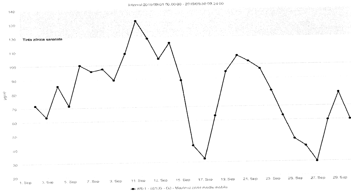
Fig. 1.2.4.1. Concentrațiile medii zilnice ale poluantului O 3
