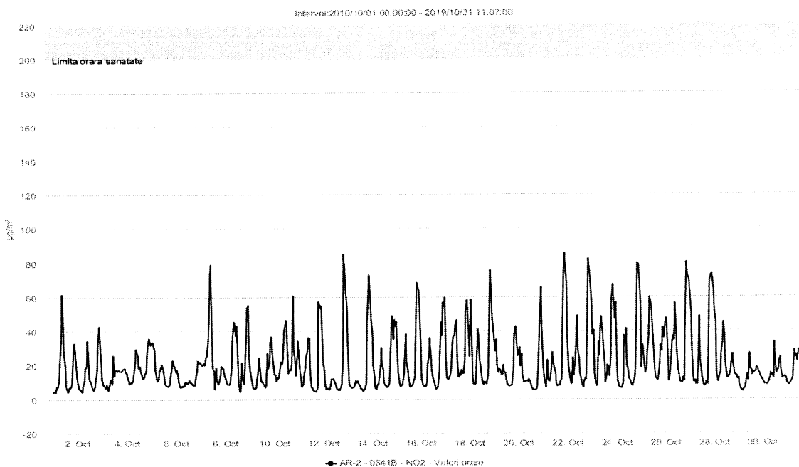
Fig.1.2.2.2. Concentrațiile medii orare ale poluantului NO 2
