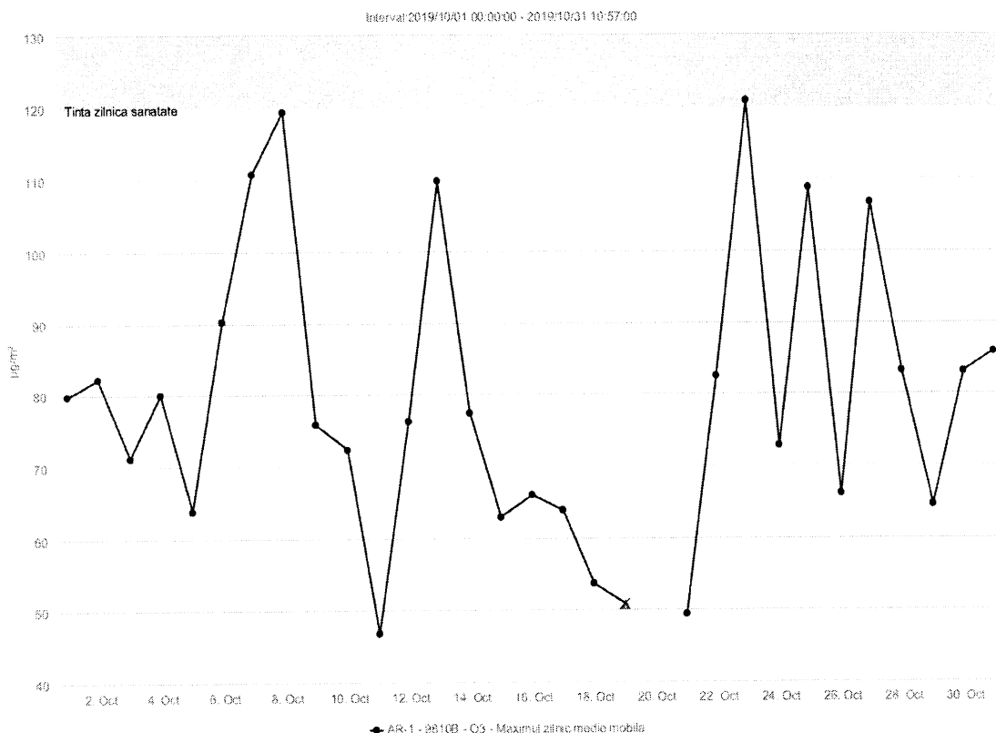
Fig. 1.2.4.1. Concentrațiile medii zilnice ale poluantului \text{O}_3
