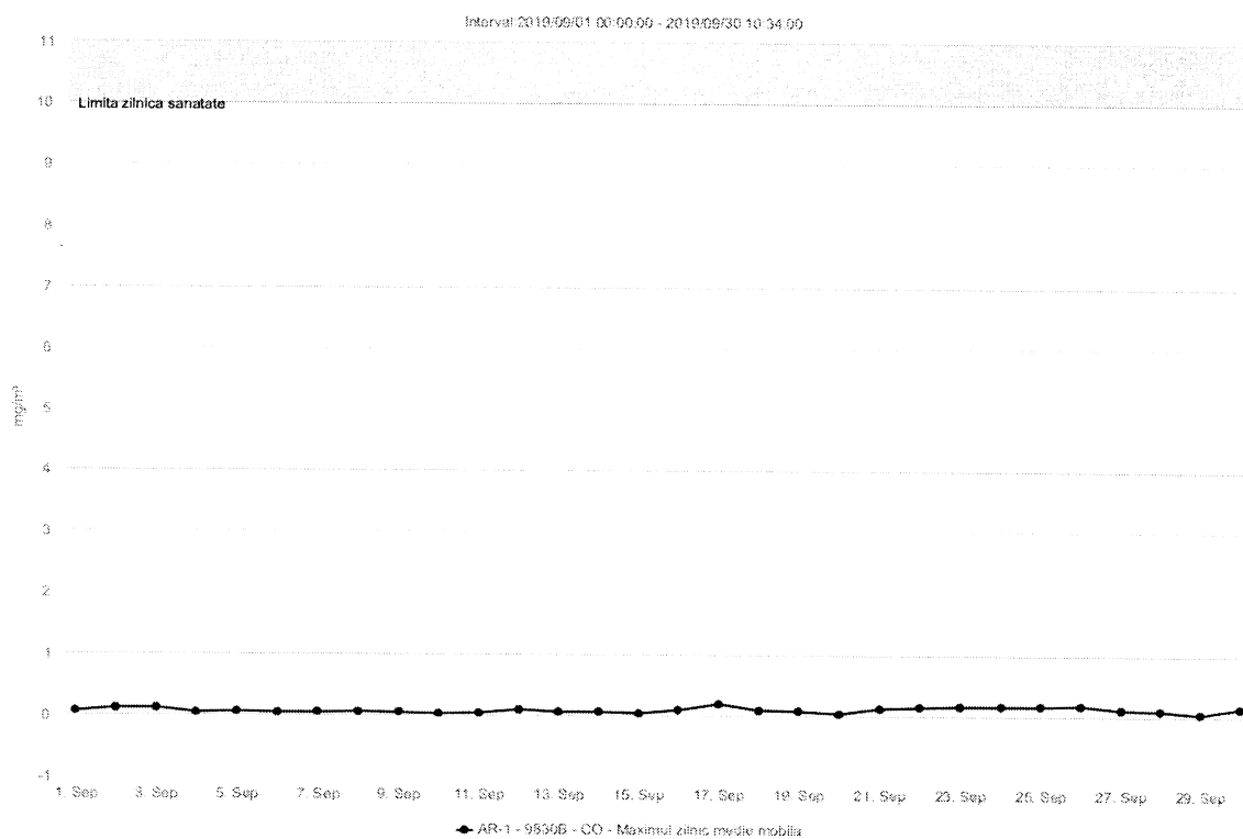
Fig. 1.2.3.2. Concentrațiile medii orare ale poluantului CO
