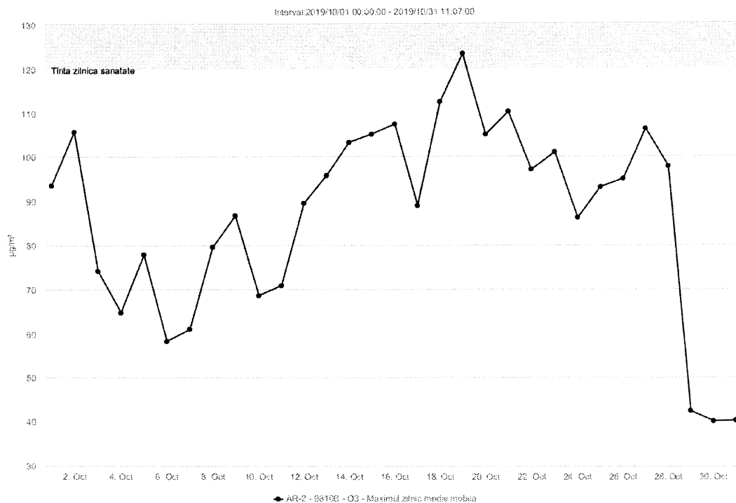
Fig. 1.2.4.2. Concentrațiile mediilor zilnice ale poluantului O 3
