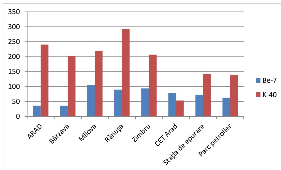
Fig. IX.1.4.1 Concentrația ^{40}\text{K} și ^7\text{Be} în probele de vegetație recoltate în județul Arad ( \text{Bq.Kg}^{-1} ).
