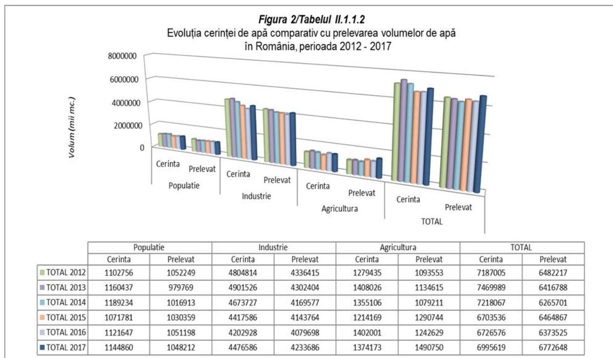
Fig. II.1.1.2.1. Evoluția cerinței de apă comparativ cu prelevarea volumelor de apă (mii m 3 )
