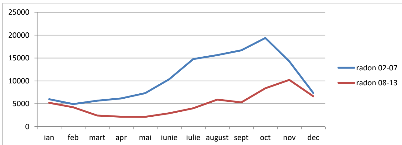
Fig. IX.1.1.4 Variația activității specifice medii lunare a radonului din atmosferă în funcție de variația diurnă( Bq\cdot m^{-3} ).
