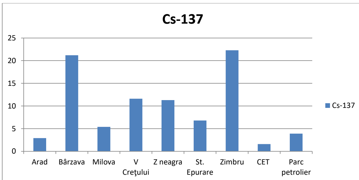
Fig. IX.1.3.1 Concentrația 137 Cs în probe de sol (BqKg -1 )
