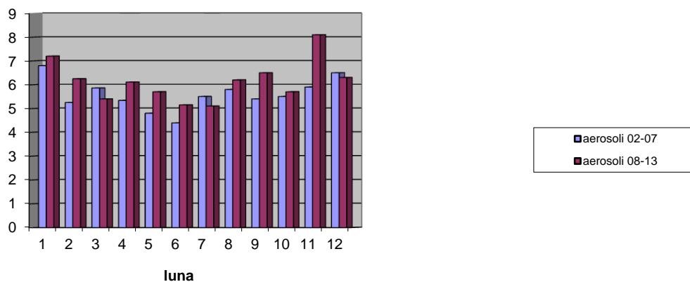
Fig. IX.1.1.3 Variația medie lunară a activității beta globale a aerosolilor atmosferici ( mBq\cdot m^{-3} ) în funcție de variația diurnă - măsurare la 5 zile
