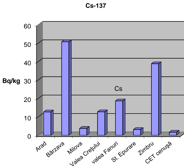
Fig. IX.1.3.1 Concentrația 137 Cs în probe de sol (BqKg -1 )
