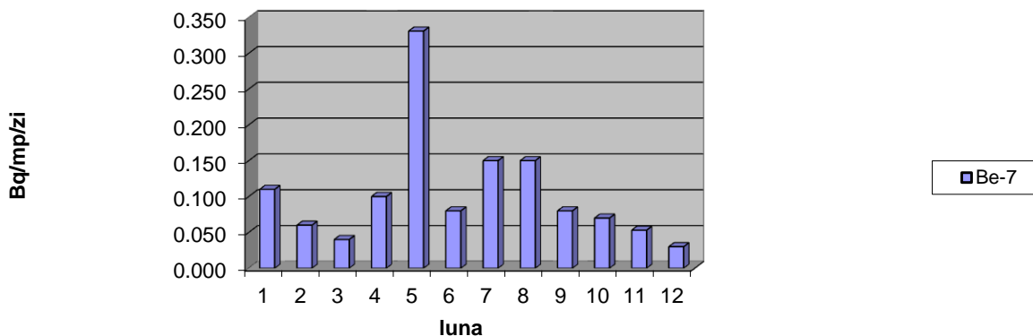
Fig IX.1.1.12 Variațiile medii lunare ale izotopului natural Be^7 în probele de depuneri lunare ( Bq \cdot m^{-2} \cdot zi^{-1} ).
