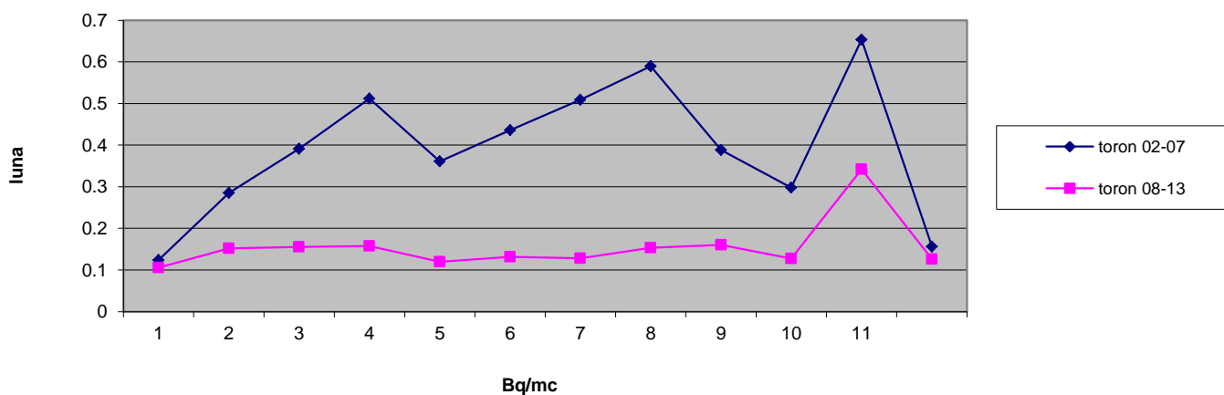
Fig. IX.1.1.5 Variația activității specifice medii lunare a toronului din atmosferă în funcție de variația diurnă (Bqm -3 ).
