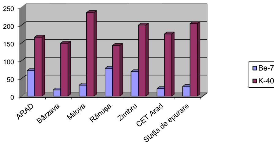
Fig. IX.1.4.1 Concentrația ^{40}\text{K} și ^7\text{Be} în probele de vegetație recoltate în județul Arad ( \text{Bq.Kg}^{-1} ).
