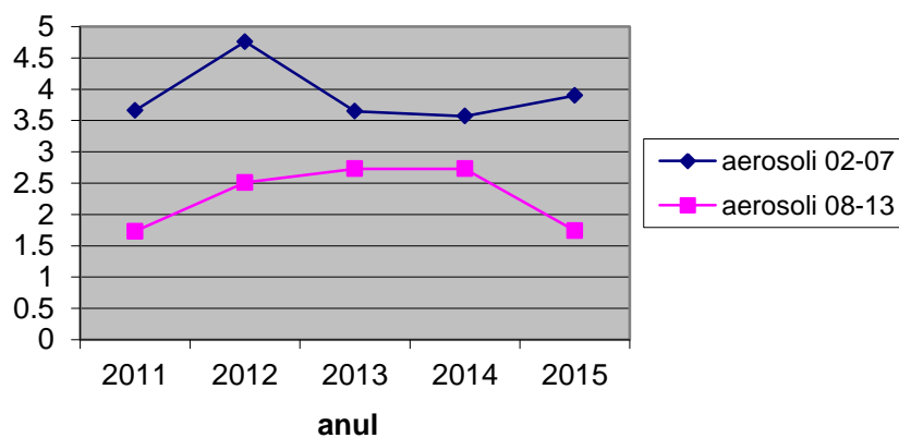
Fig. IX.1.1.3 Variația medie lunară a activității beta globale a aerosolilor atmosferici ( mBq\cdot m^{-3} ) în funcție de variația diurnă - măsurare la 5 zile
