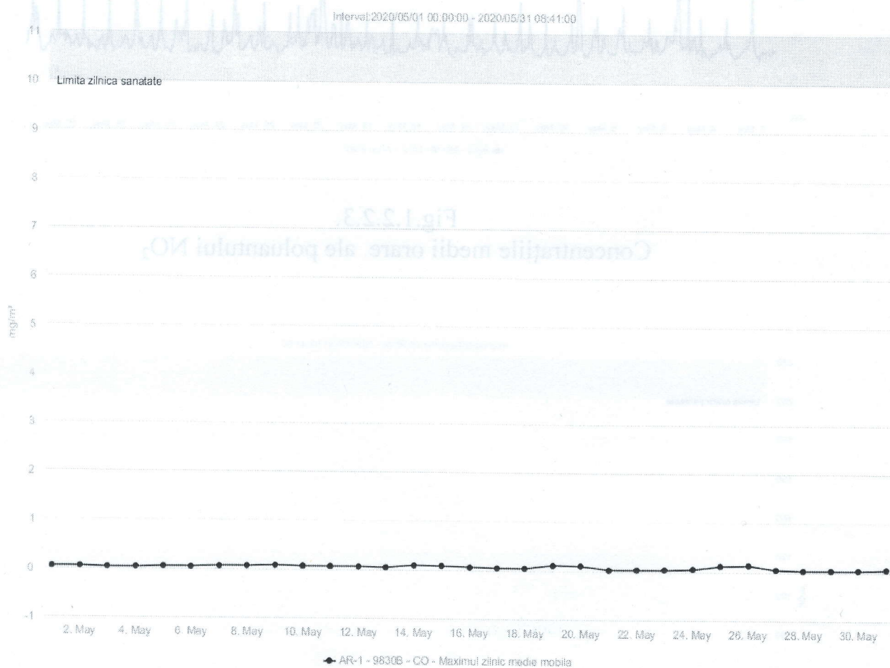
Fig. 1.2.3.1. Concentrațiile medii orare ale poluantului CO
