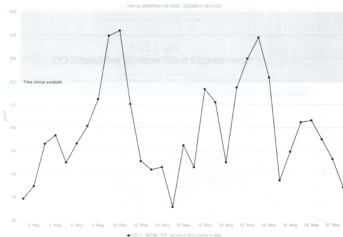
Fig. 1.2.4.2. Concentrațiile mediilor zilnice ale poluantului \text{O}_3
