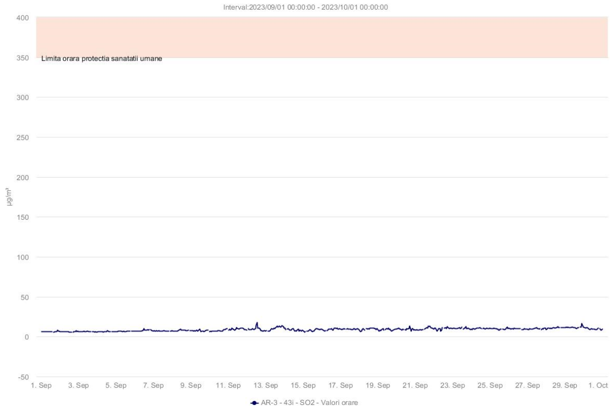
Fig. 1.2.1.5. Concentrațiile medii orare ale poluantului SO 2
