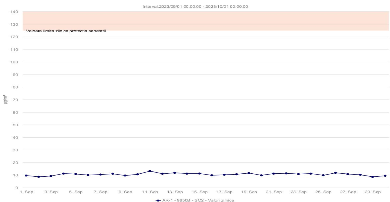
Fig. 1.2.1.2. Concentrațiile medii zilnice ale poluantului SO 2
