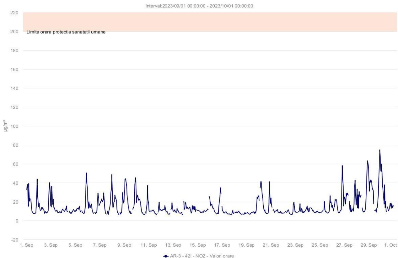
Fig.1.2.2.3. Concentrațiile medii orare ale poluantului NO 2
