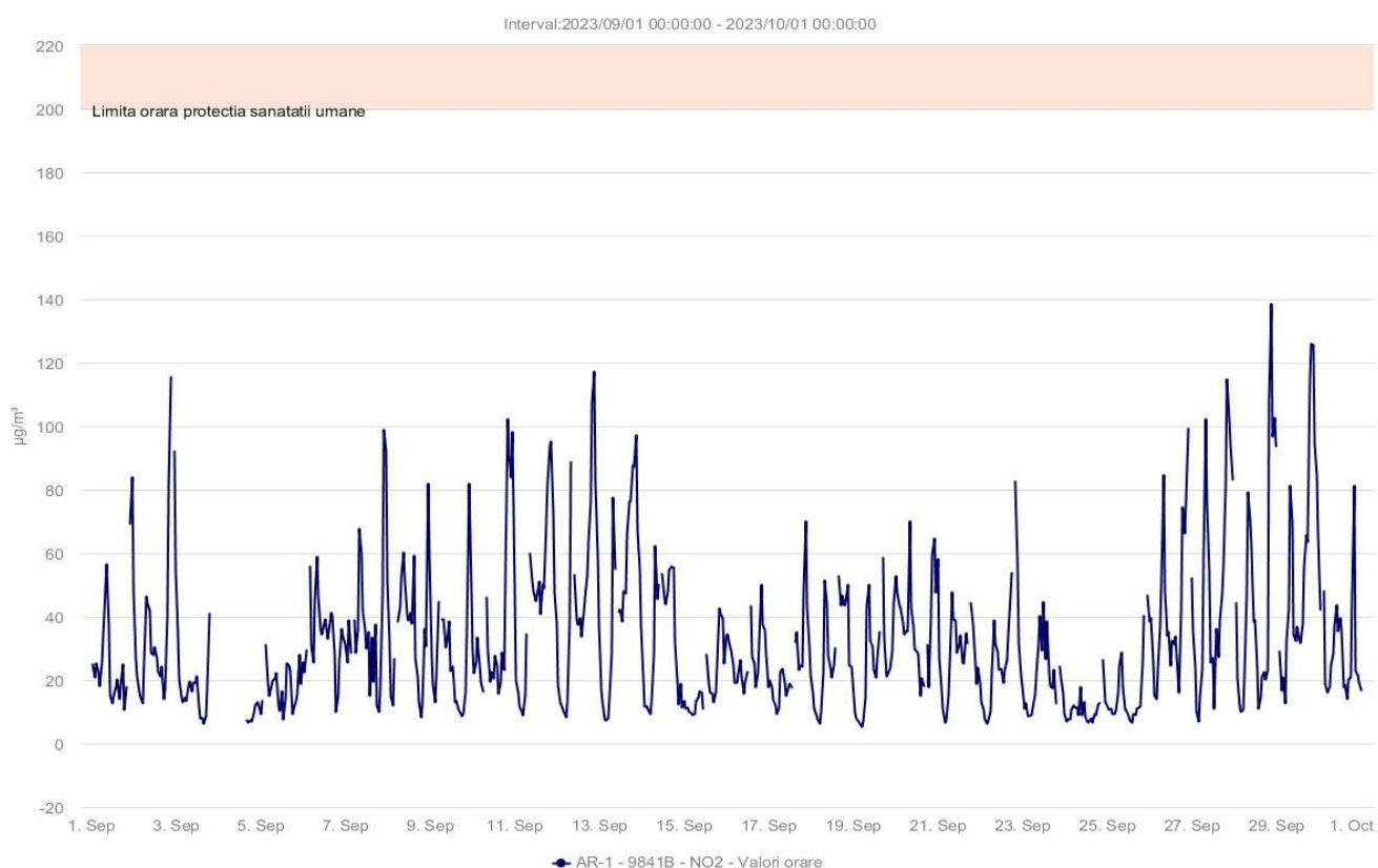
Fig.1.2.2.1. Concentrațiile medii orare ale poluantului \text{NO}_2
