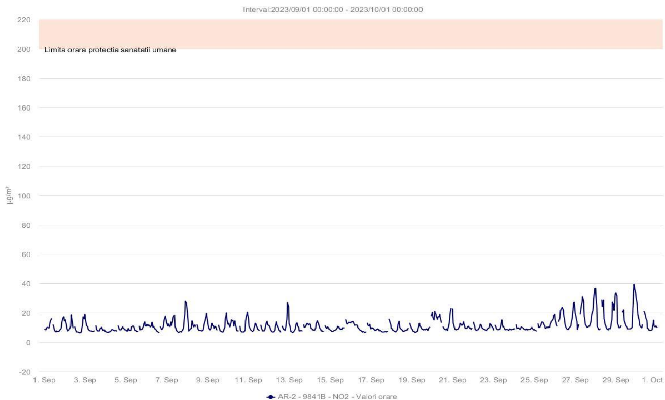
Fig.1.2.2.3. Concentrațiile medii orare ale poluantului NO 2
