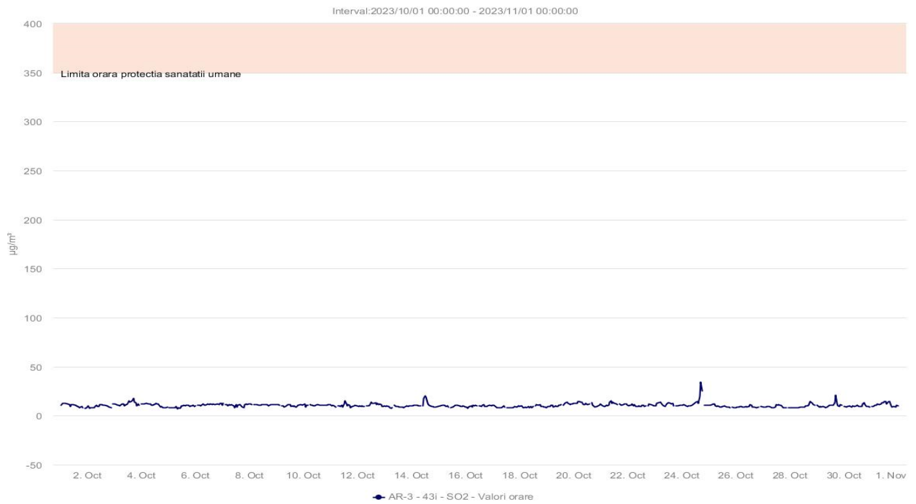
Fig. 1.2.1.5. Concentrațiile medii orare ale poluantului SO 2
