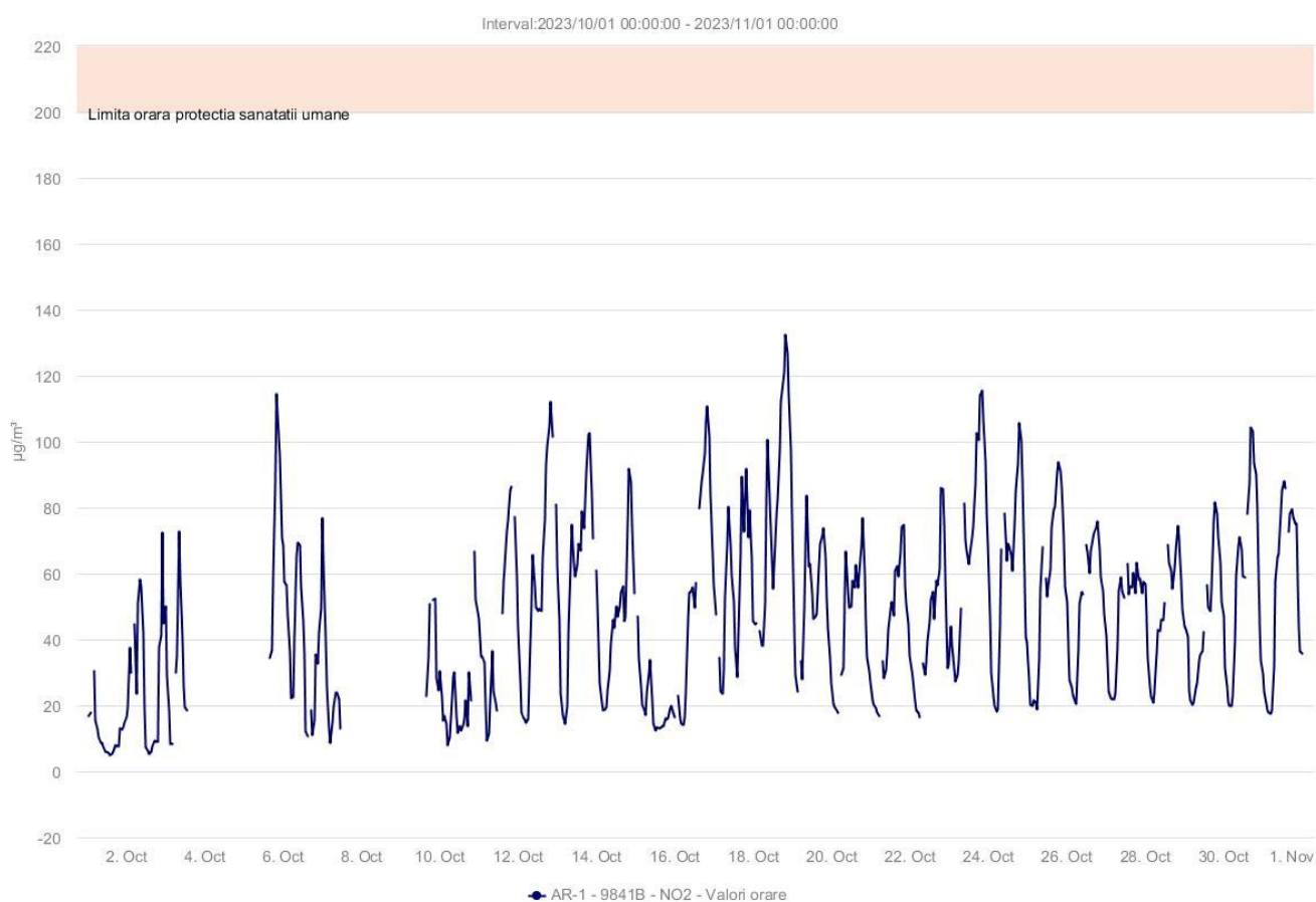
Fig.1.2.2.1. Concentrațiile medii orare ale poluantului \text{NO}_2
