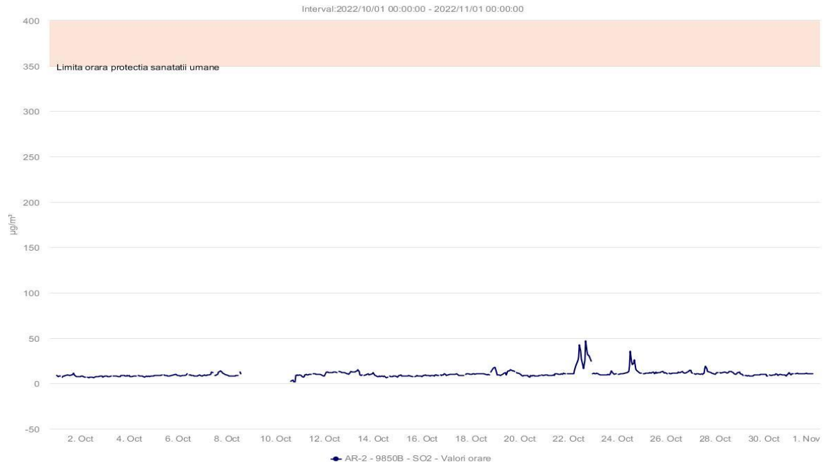
Fig. 1.2.1.4. Concentrațiile medii zilnice ale poluantului SO 2
