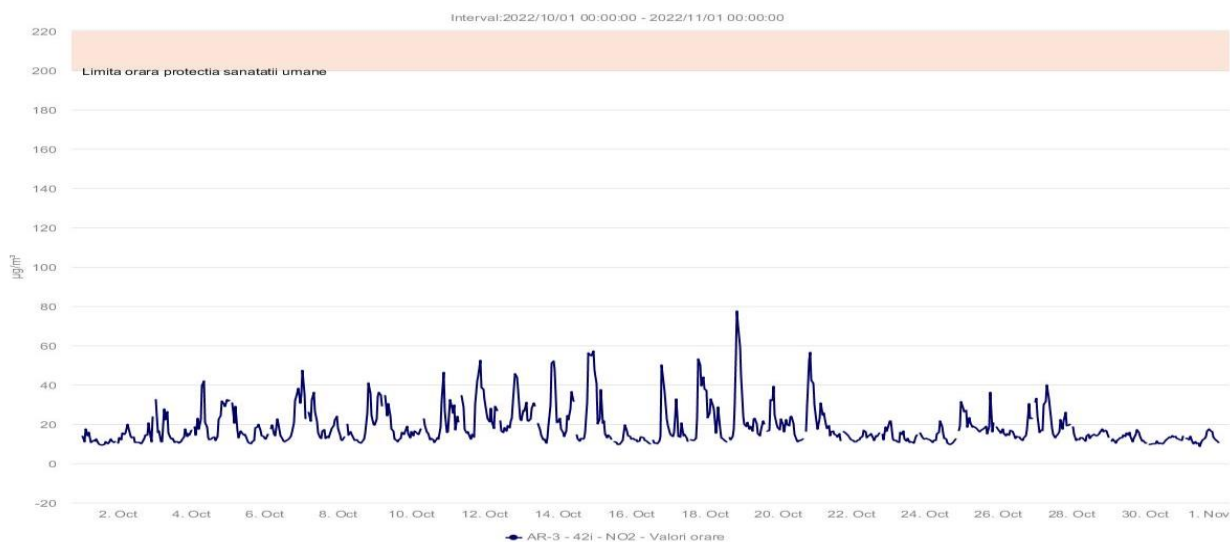
Fig.1.2.2.3. Concentrațiile medii orare ale poluantului NO 2
