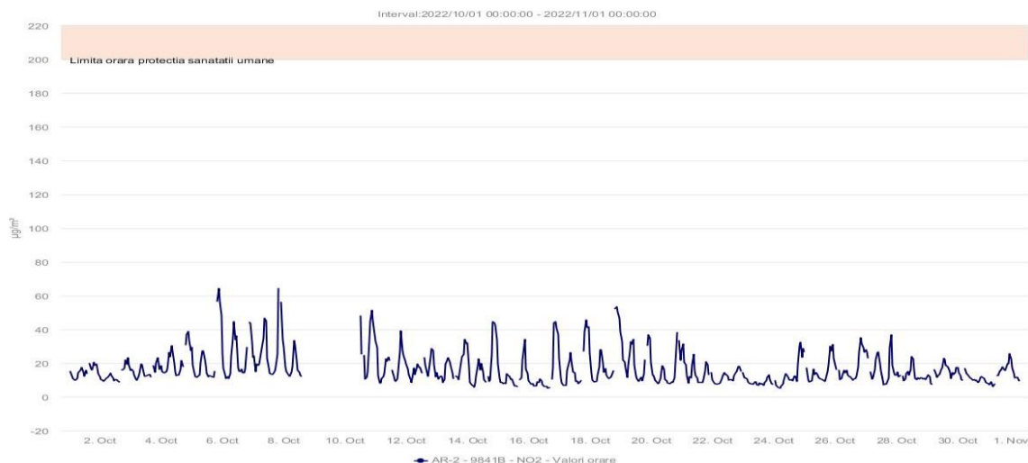
Fig.1.2.2.2. Concentrațiile medii orare ale poluantului \text{NO}_2
