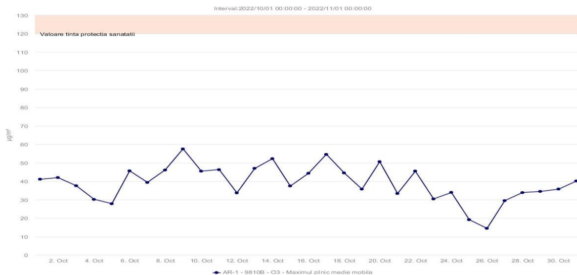
Fig. 1.2.4.1. Concentrațiile medii zilnice ale poluantului \text{O}_3
