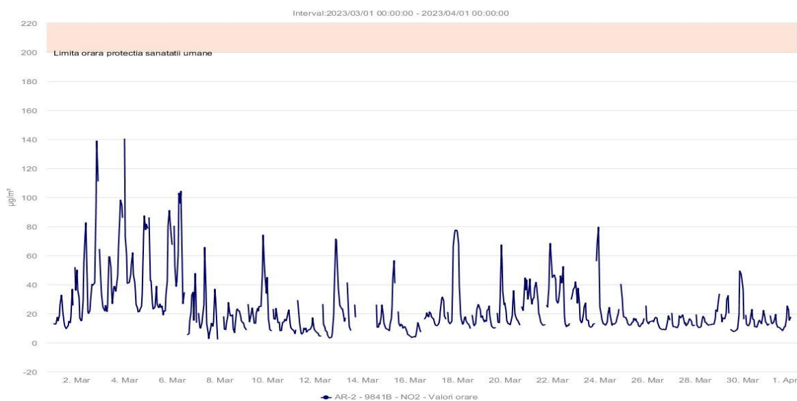
Fig.1.2.2.2. Concentrațiile medii orare ale poluantului \text{NO}_2
