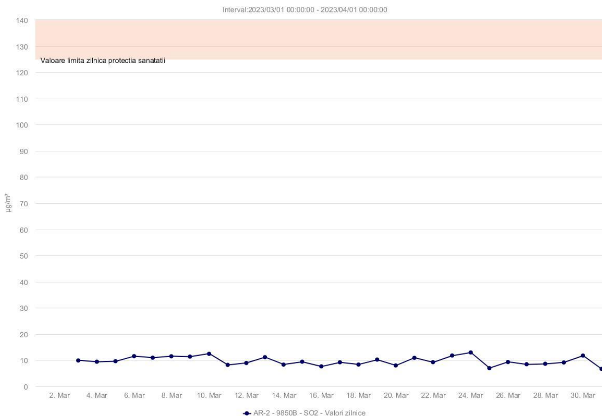
Fig. 1.2.1.4. Concentrațiile medii zilnice ale poluantului SO 2
