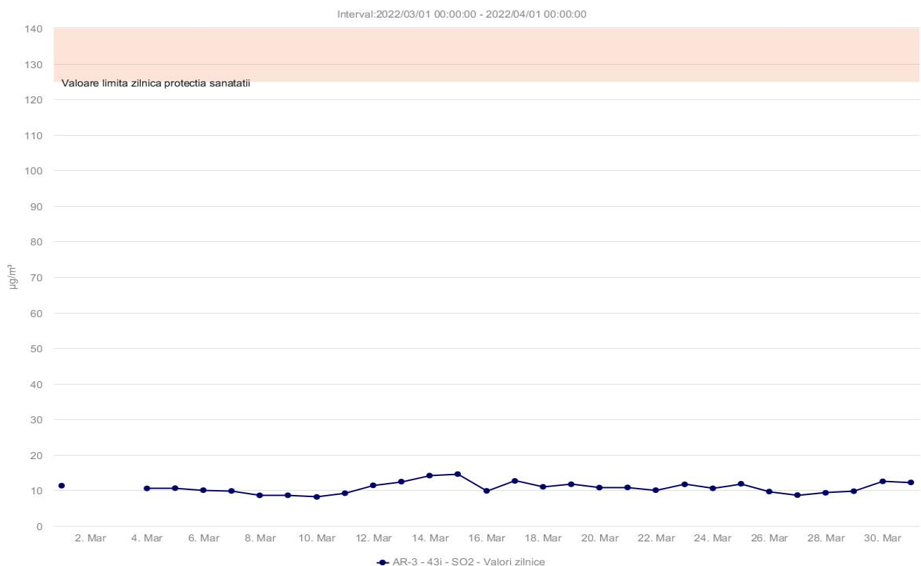
Fig. 1.2.1.6. Concentrațiile medii zilnice ale poluantului SO 2
