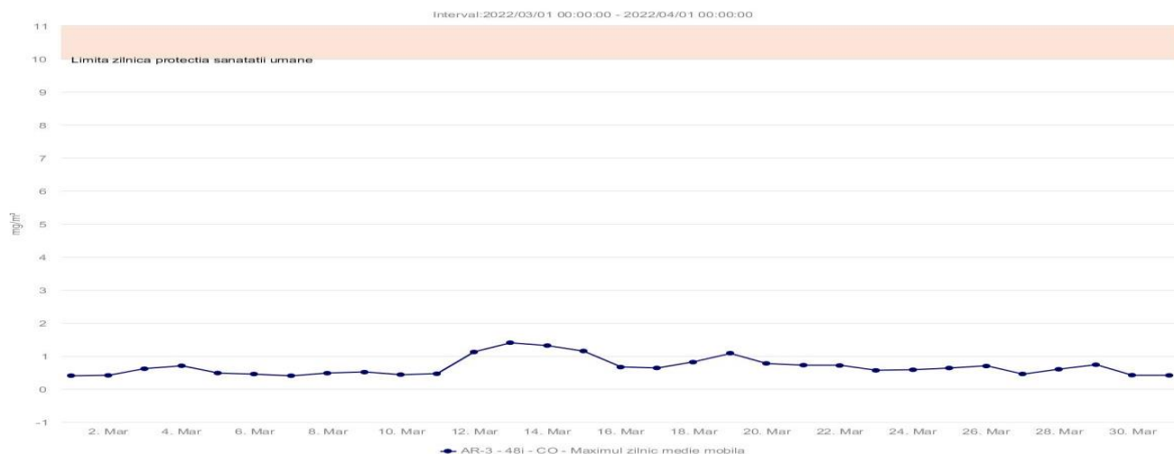
Fig. 1.2.3.3. Concentrațiile medii orare ale poluantului CO
