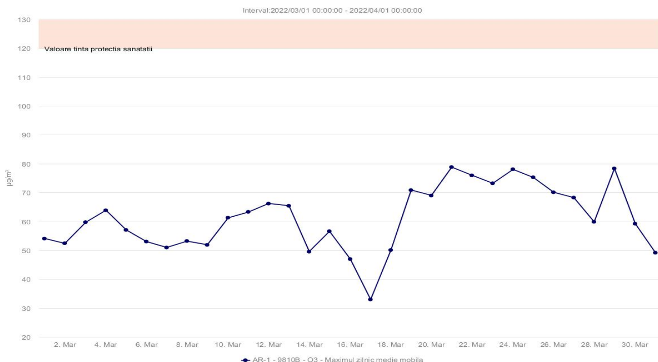
Fig. 1.2.4.1. Concentrațiile medii zilnice ale poluantului \text{O}_3
