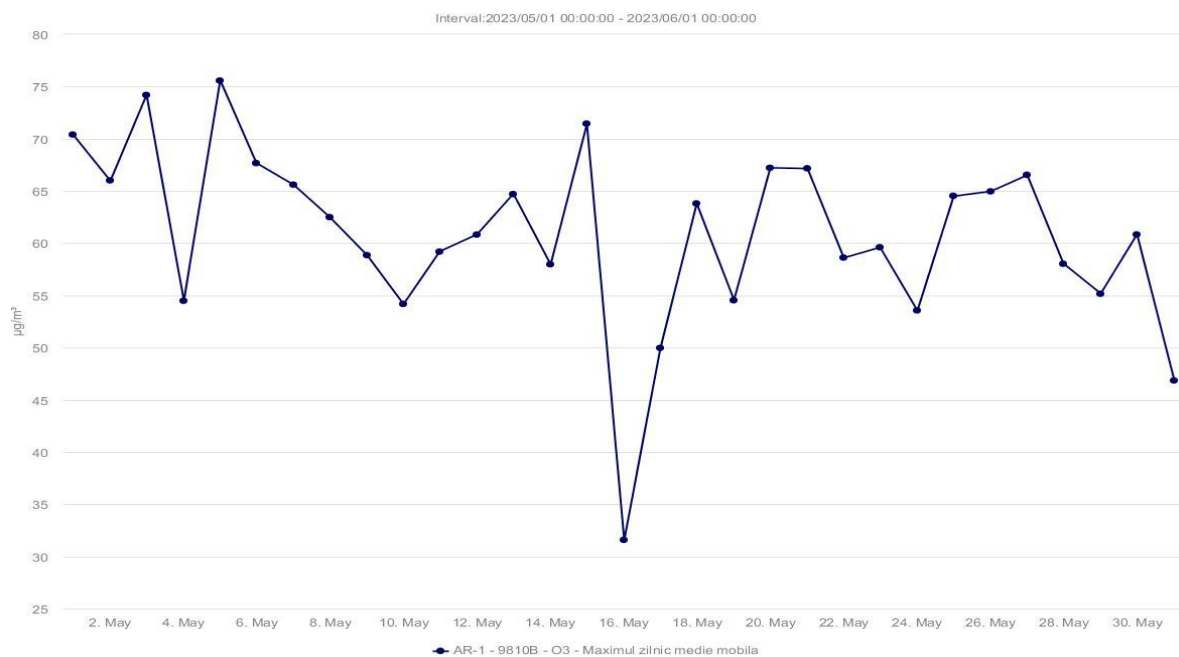
Fig. 1.2.4.1. Concentrațiile medii zilnice ale poluantului \text{O}_3
