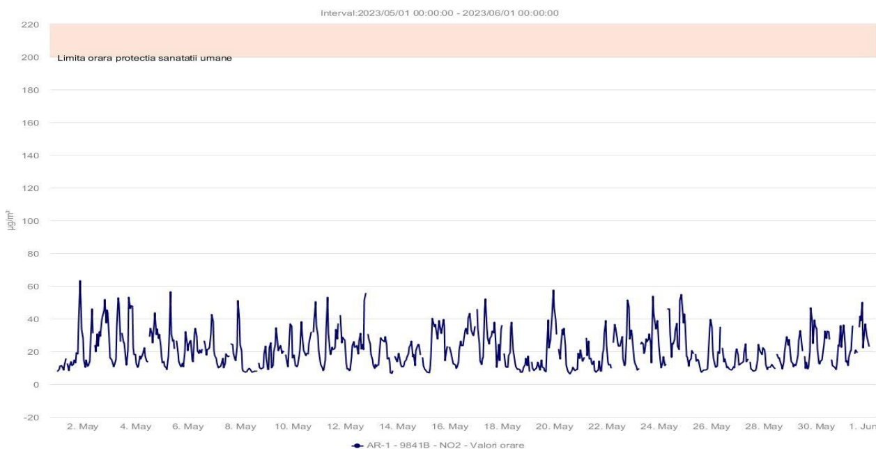
Fig.1.2.2.1. Concentrațiile medii orare ale poluantului \text{NO}_2
