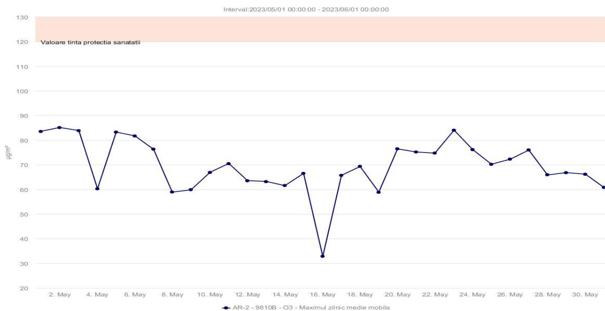
Fig. 1.2.4.2. Concentrațiile mediilor zilnice ale poluantului O 3
