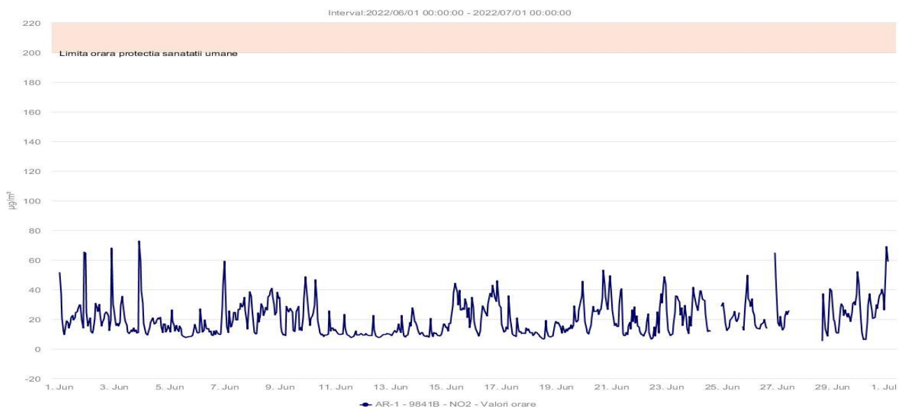
Fig.1.2.2.1. Concentrațiile medii orare ale poluantului \text{NO}_2
