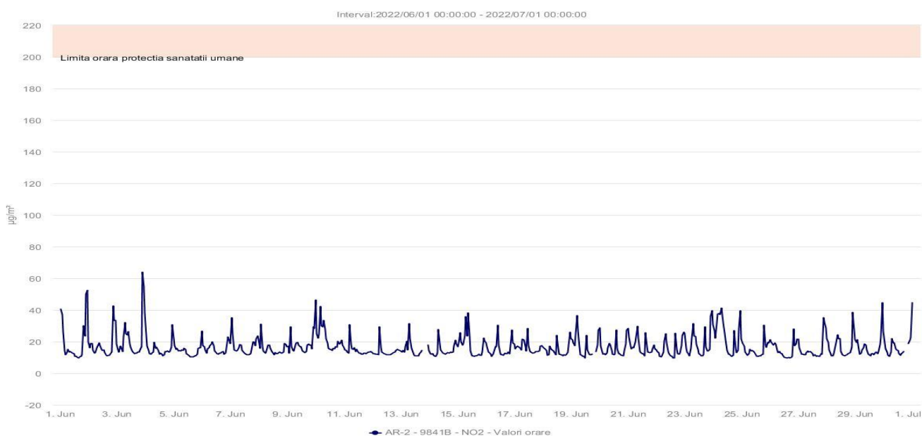
Fig.1.2.2.2. Concentrațiile medii orare ale poluantului \text{NO}_2
