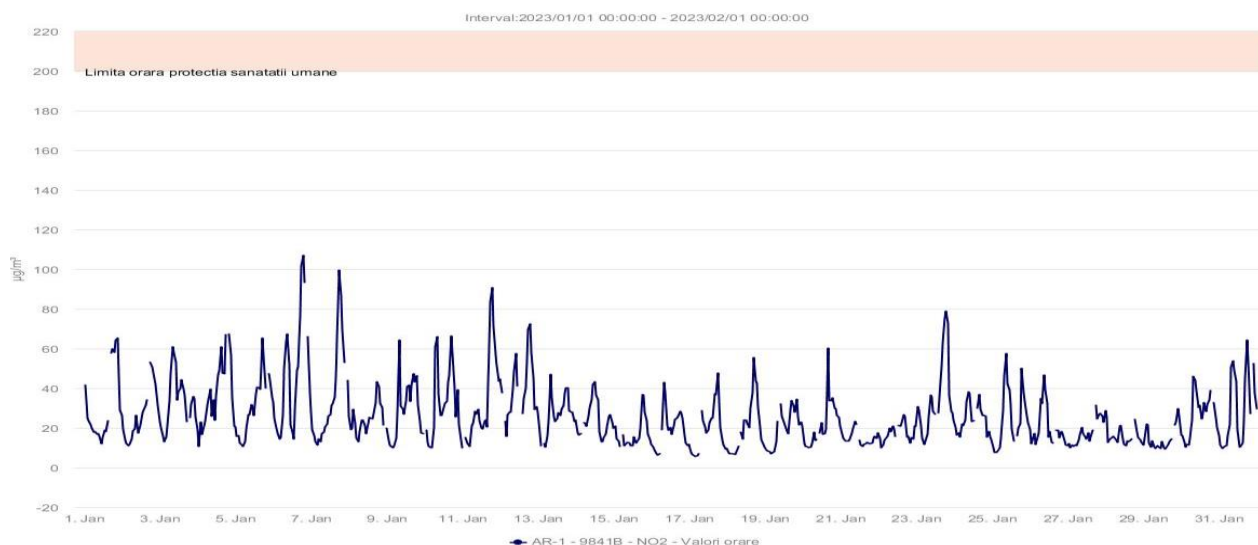
Fig.1.2.2.1. Concentrațiile medii orare ale poluantului \text{NO}_2
