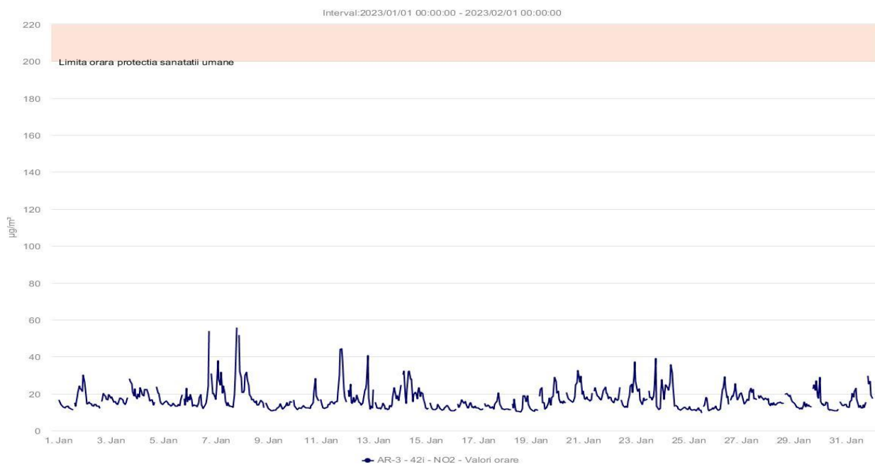
Fig.1.2.2.3. Concentrațiile medii orare ale poluantului NO 2
