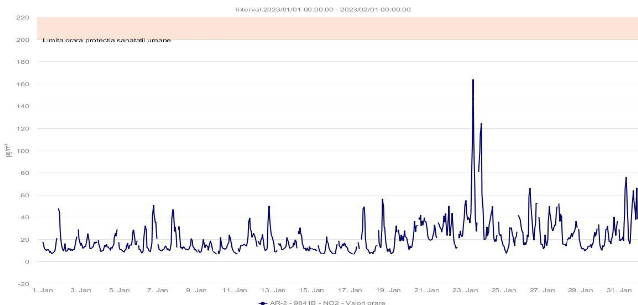
Fig.1.2.2.2. Concentrațiile medii orare ale poluantului \text{NO}_2
