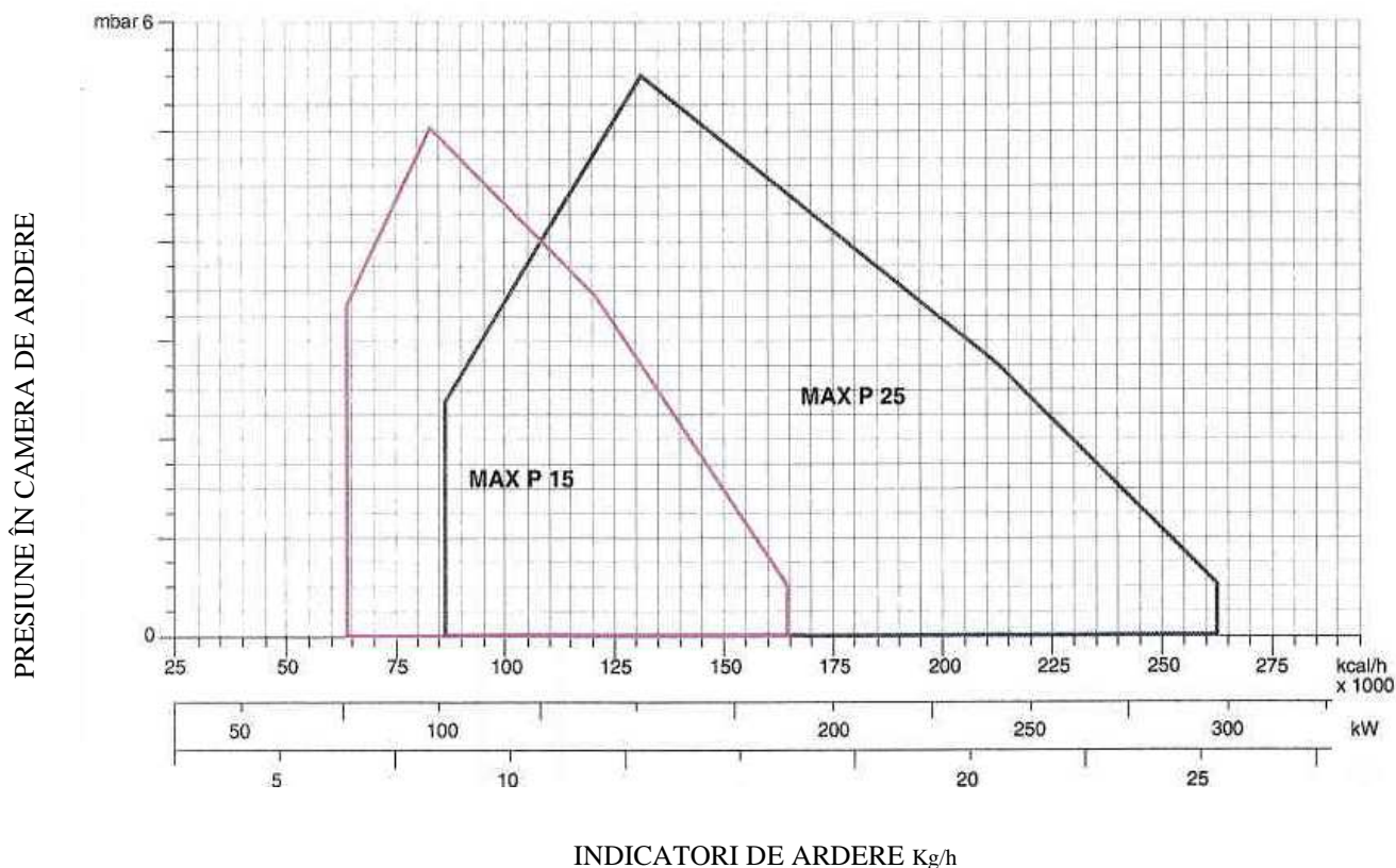
Figură 4: curbele de performanță ale arzătoarelor
