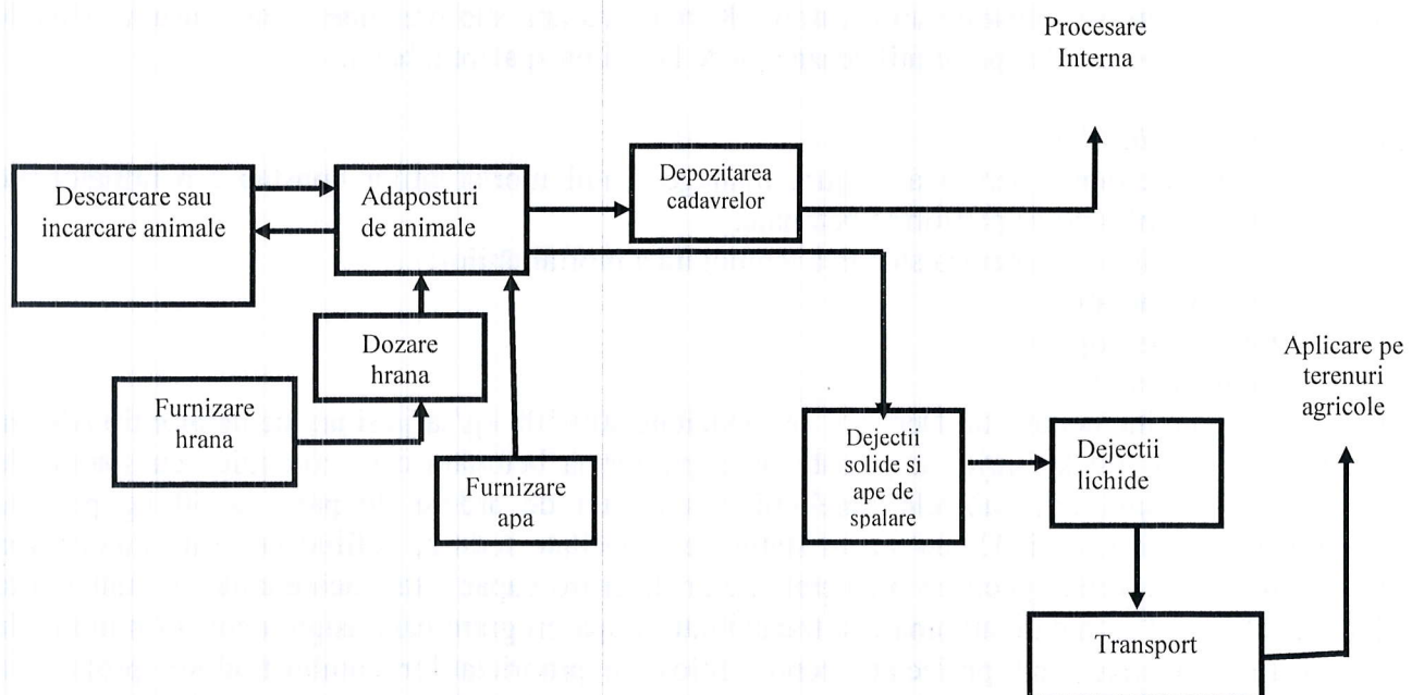
Figura 8.2.1.: Schema fluxului tehnologic
