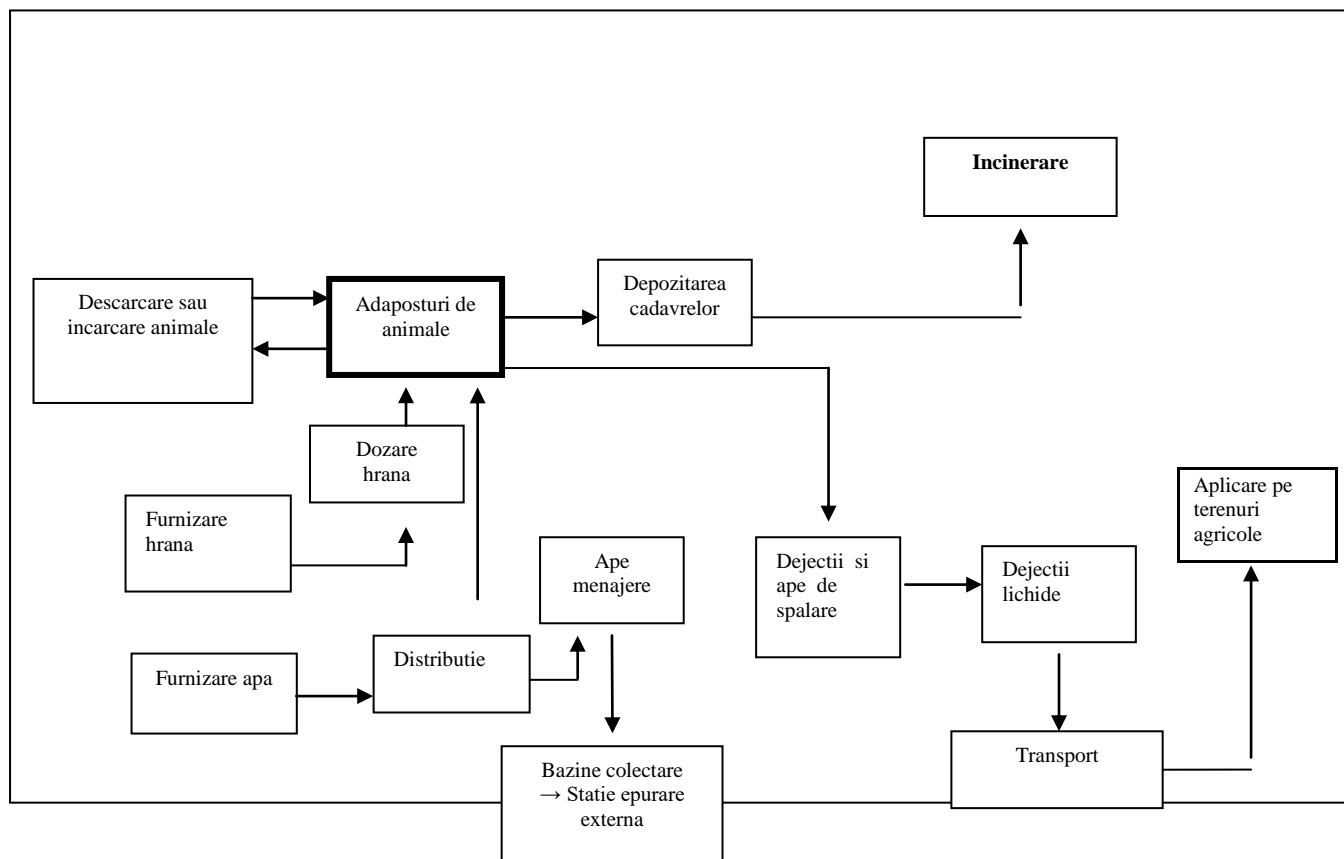
Figura 8.2.1.: Schema fluxului tehnologic
