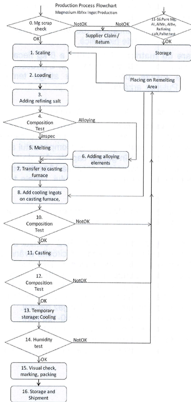
Fig. 1 Schema procesului de reciclare deșeurii magneziu
